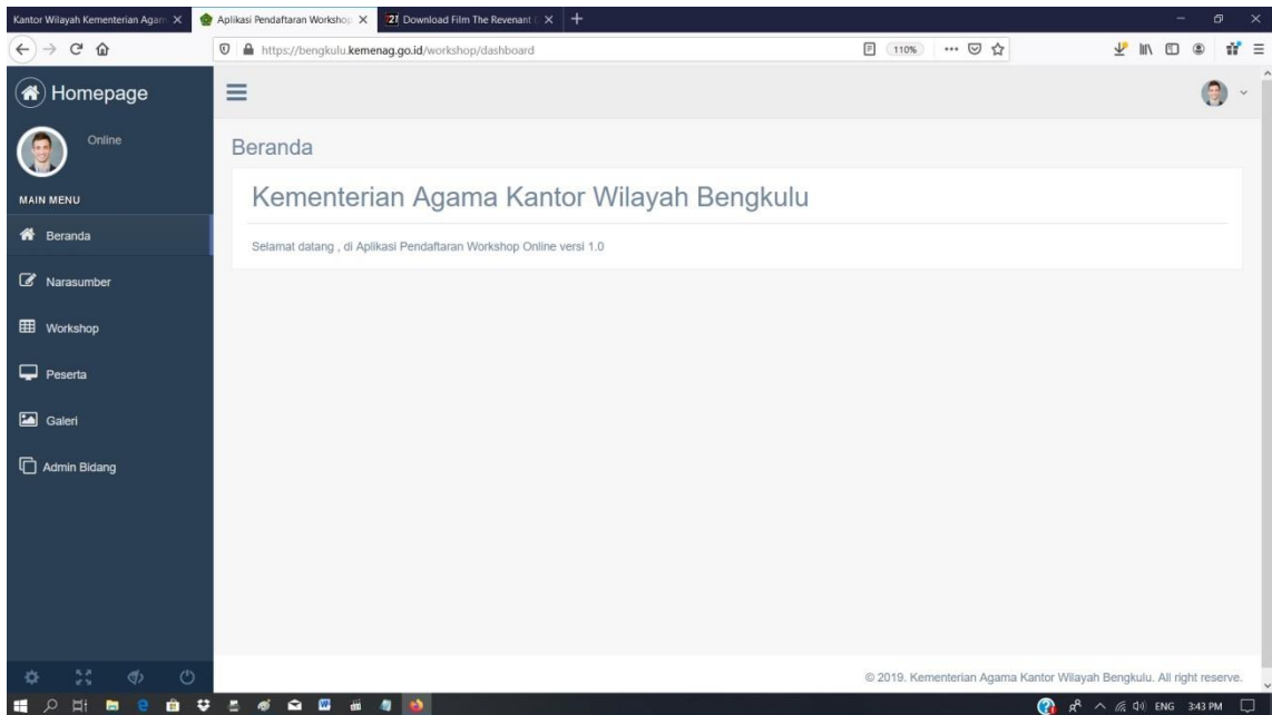
Halaman Beranda
