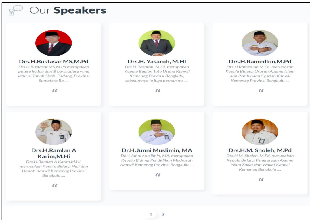
Halaman Narasumber
