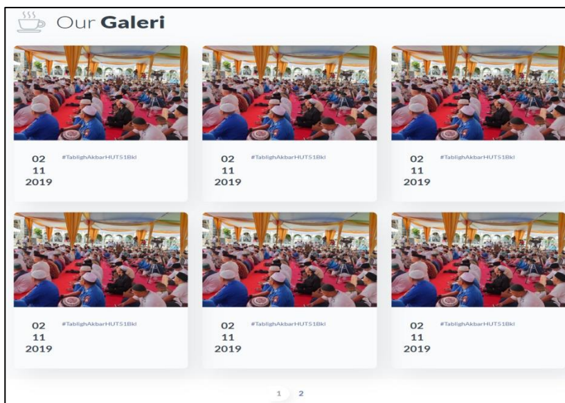
Halaman Galeri
