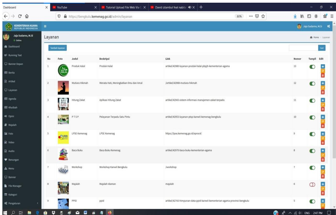
Menu Layanan
